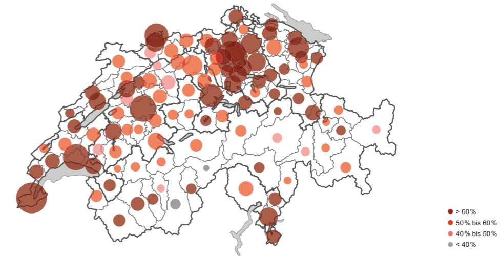
Abb. 7.5.2.3 Heatmap Mehrfamilienhäuser (2018)
